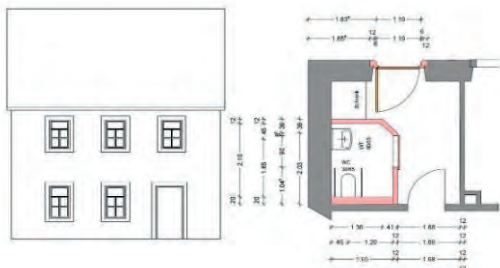
Planung eines barrierefreien Zugangs und eines barrierefreien WCs in der „Alten Schule“. Der Zugang wäre vom Kirchplatz her möglich
